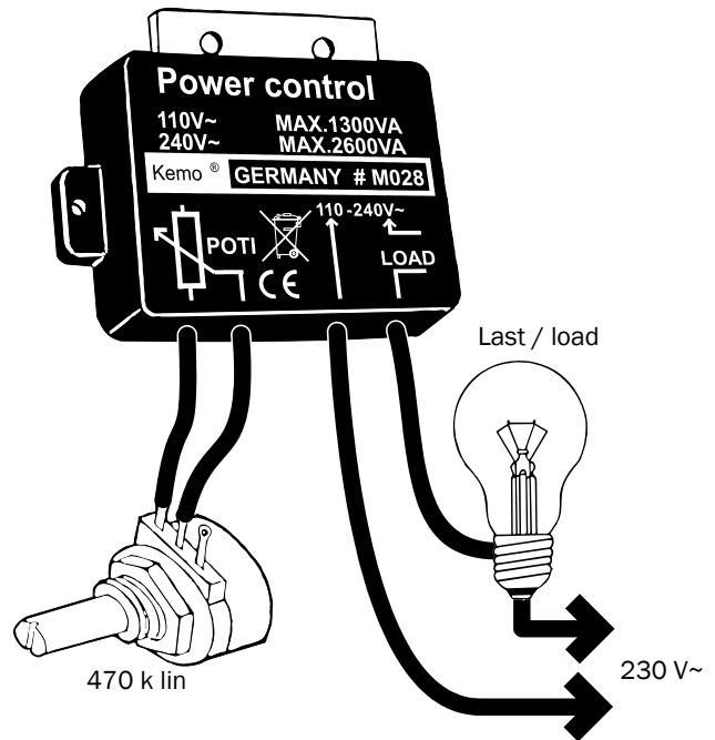
Betrieb des Moduls mit einem Poti 470 k lin. Operation of the modul with a poti 470 k lin.
