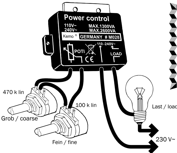
Betrieb des Moduls mit 2 Potis (1 Grob- und 1 Feinregler). Potis: 470 k + 100 k lin. Operating of the module with 2 potis' (1 coarse and 1 fine control). Potis': 470 k + 100 k lin.
